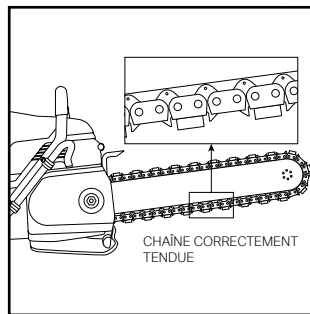
Réglage simple de la tension de la chaîne
